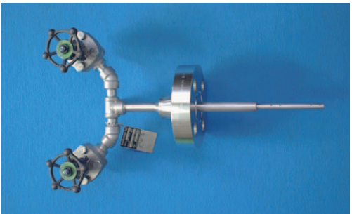
同社の代表製品であるバーフローチューブ（差圧式ピトー管）
